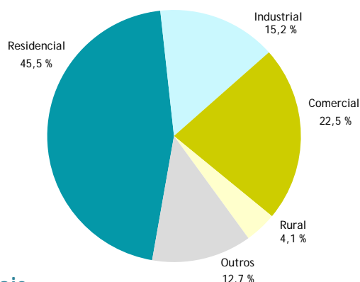
Receita de Energia por Classe de Consumidores
